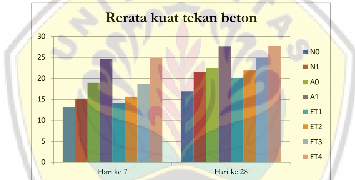
Gambar 2. Data hasil rerata kuat tekan beton umur 7 dan 28 hari
