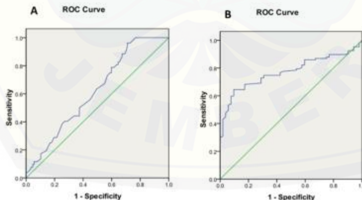
Gambar 1. Kurva ROC A. MPV, B. Leukosit
