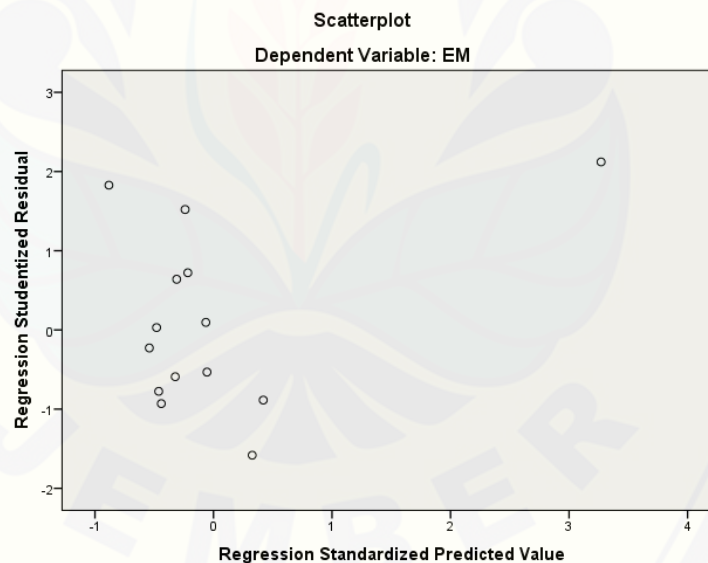
Gambar 1. Hasil Uji Heteroskdastisitas
