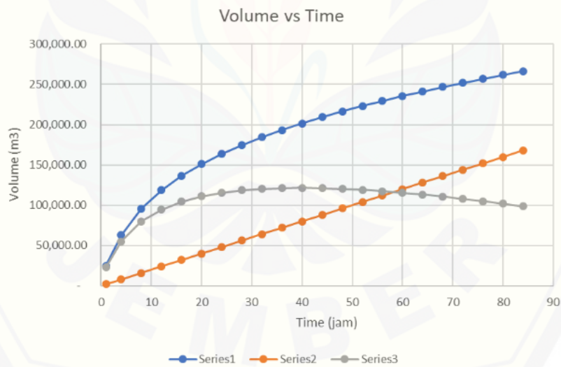
Gambar 2. Grafik Perhitungan Volume Optimum Sump berbanding Waktu di Pit Barat
