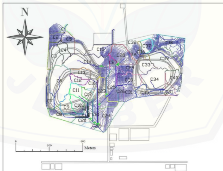
Gambar 1. Keseluruhan Catchment Area pada Topografi
