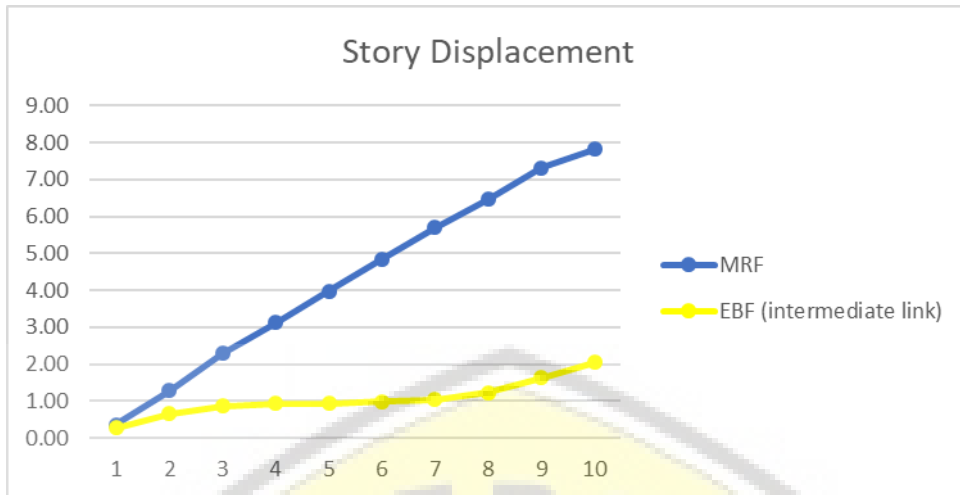
Gambar 3. Nilai Story Displacement MRF dan EBF
