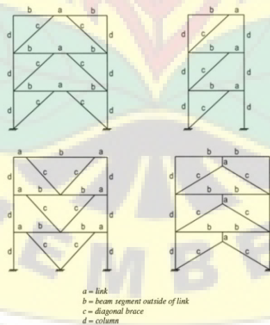
Gambar 1. Konfigurasi EBF
