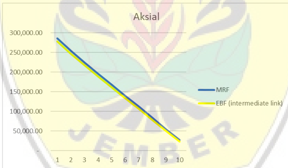
Gambar 4. Perbandingan Gaya Aksial pada Kolom MRF dan EBF
