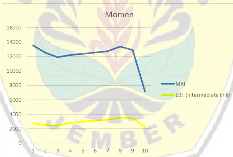
Gambar 6. Perbandingan Momen pada Balok MRF dan EBF
