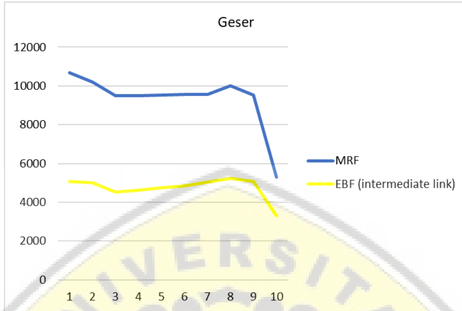
Gambar 5. Perbandingan Gaya Geser pada Balok MRF dan EBF
