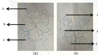
Gambar 12. Ilustrasi Dilatasi pada Batik Gajah Oling
