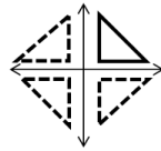
Refleksi terhadap sumbu-X dan Y
