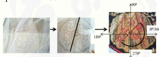
Gambar 10. Rotasi sebesar 180^\circ melalui titik asal (0,0)
