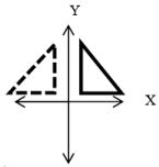
Refleksi terhadap sumbu-Y
