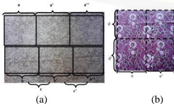
Gambar 9. Translasi pada Batik Gajah Oling
