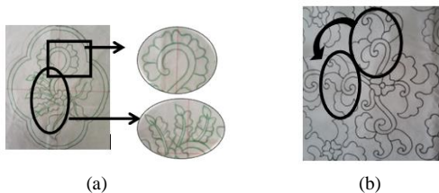
Gambar 8. Kesebangunan dan Kekongruenan pada Batik Gajah Oling
