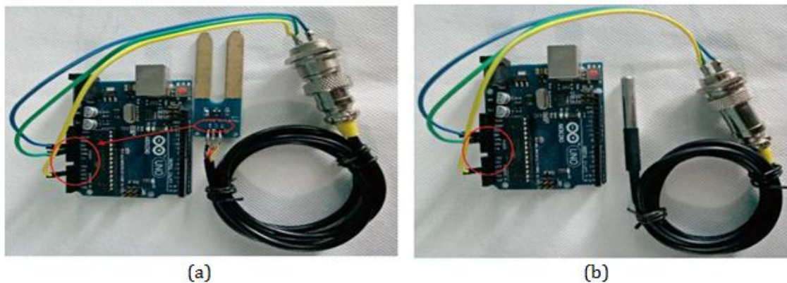
Gambar 2. Bentuk Sensor (a) Kelembaban Tanah dan (b) Suhu Tanah
