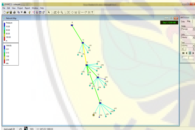
Gambar 3. Visualisasi tekanan dan kecepatan pada jaringan di distribusi air bersih PNPM Mandiri
