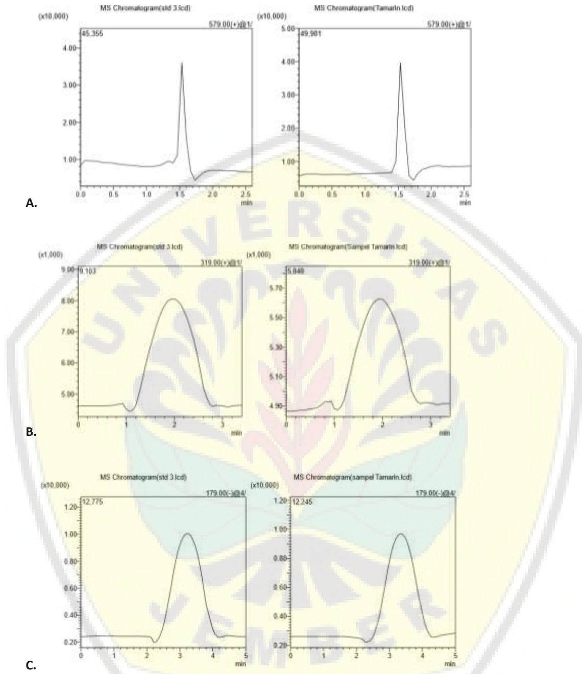
Gambar 1. Chromatogram standar dan sampel ekstrak biji Tamarindus indica .
