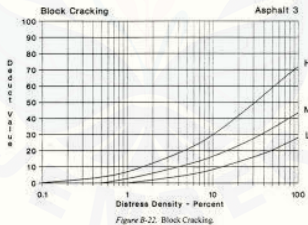
Gambar 2.20 Deduct Value Retak Kotak-kotak ( Block Cracking ) Sumber : Hardiyatmo, 2007
