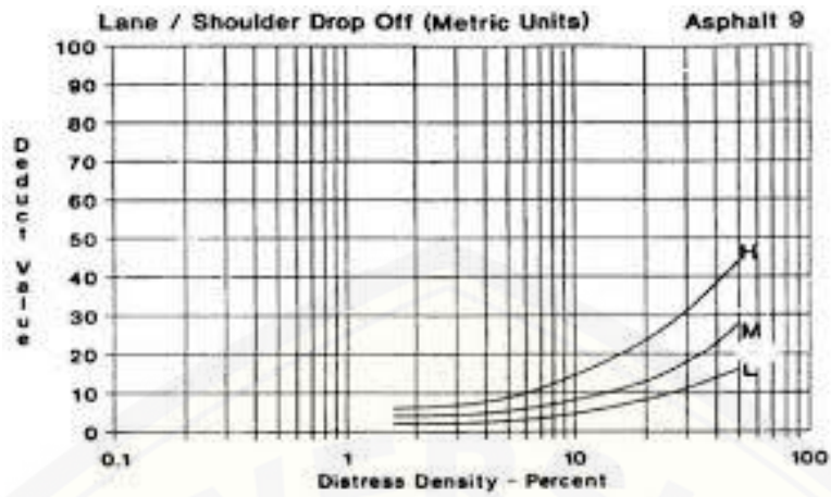
Gambar 2.23 Deduct Value Penurunan Bahu pada Jalan Sumber : Hardiyatmo, 2007
