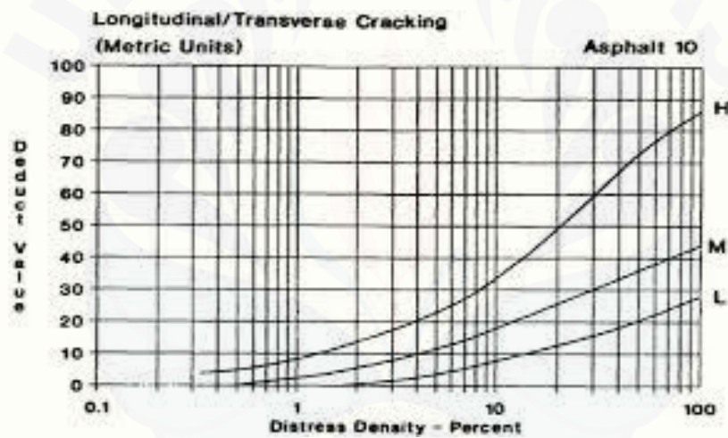
Gambar 2.24 Deduct Value Retak Memanjang dan Melintang Sumber : Hardiyatmo, 2007
