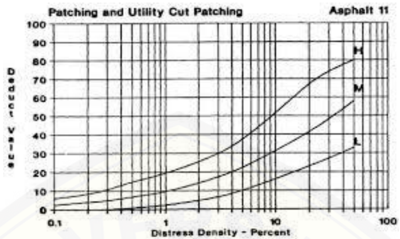
Gambar 2.25 Deduct Value Tambalan dan Galian Utilitas
