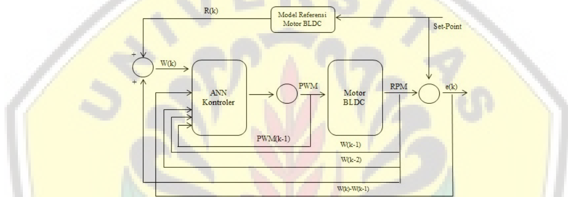
Gambar 7. Sistem Kontrol Elektronik Diferensial Kendaraan Listrik
