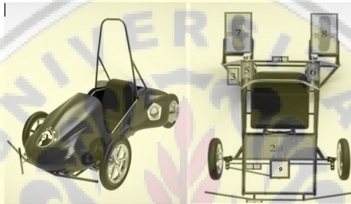
Gambar 4. Bentuk Kendaraan Listrik dengan Elektronik Diferensial
