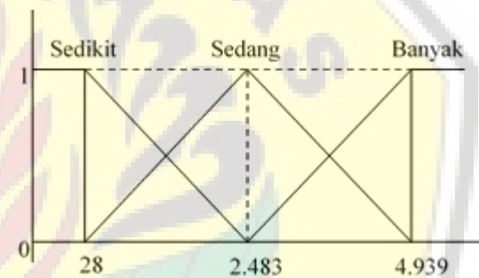
Gambar 3 Fungsi Keanggotaan Variabel Stok
