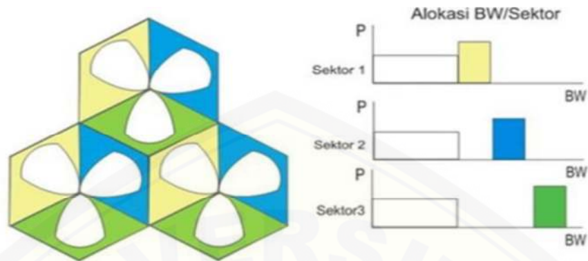
Gambar 2.7 Fractional Frekuensi Reuse (Sumber: Usman,U.K, dkk, 2011)
