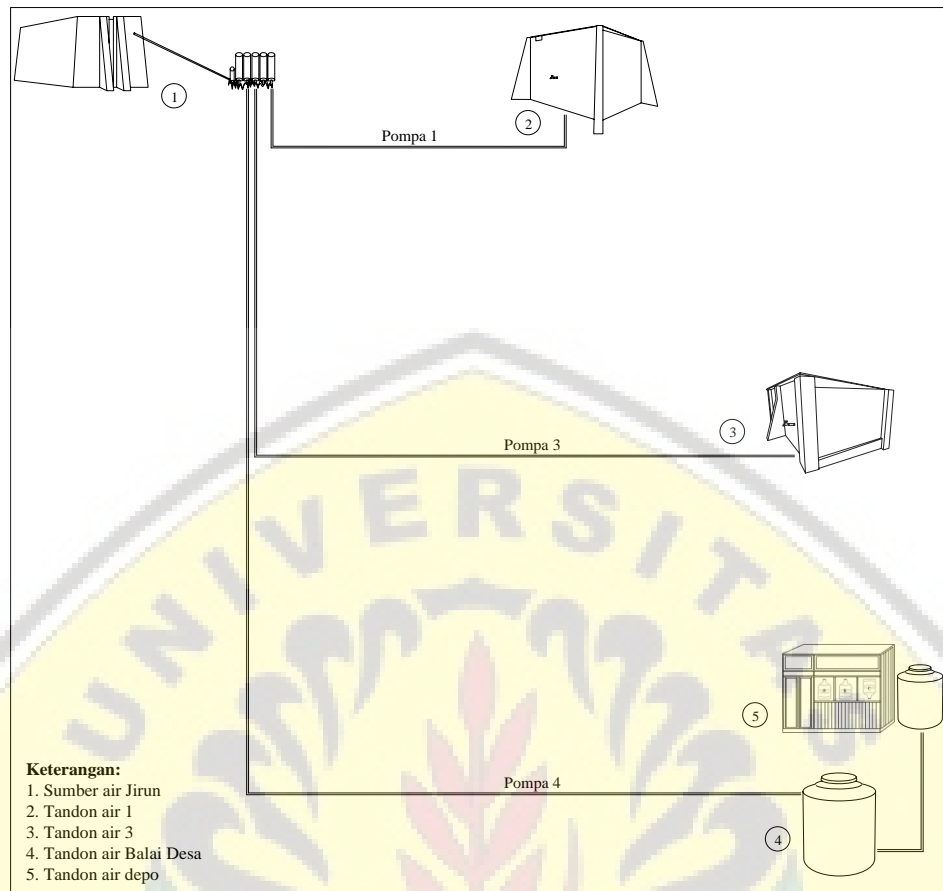
Gambar 10. Skema distribusi air bersih Subsistem 1
