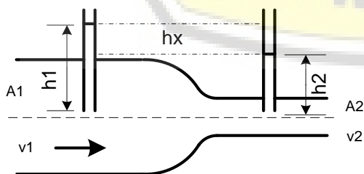
Gambar 4. Venturimeter terbuka
