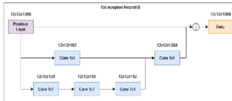
Gambar 2. 10 Inception Resnet B (Sumber : Ejournal Universitas majalengka )
