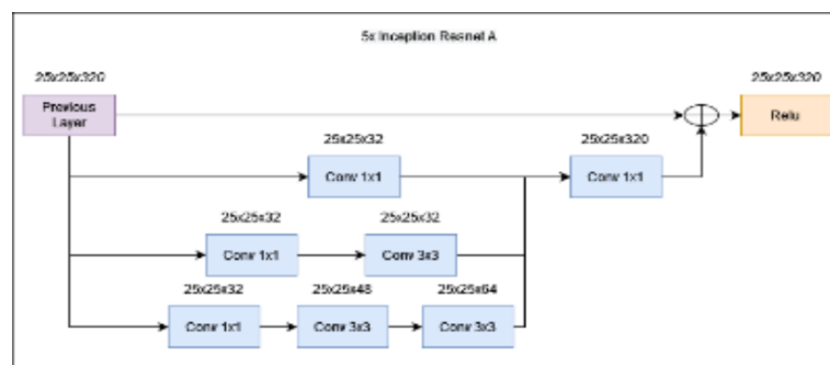
Gambar 2. 9 Inception Resnet A (Sumber : Ejournal Universitas majalengka )
