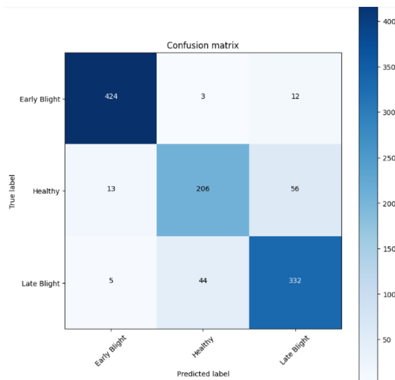
Gambar 4. 10 Confusion Matrix Arsitektur Inception ResnetV2 dengan pembagian data 70:30
