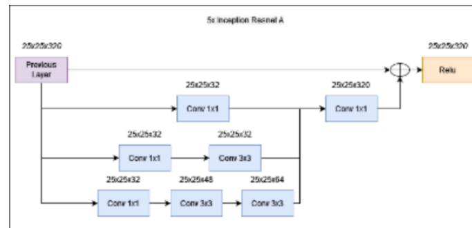
Gambar 2. 12 Reduction A (Sumber : Ejournal Universitas majalengka)
