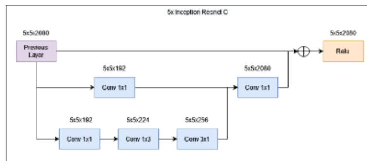
Gambar 2. 11 Inception Resnet C (Sumber : Ejournal Universitas majalengka )
