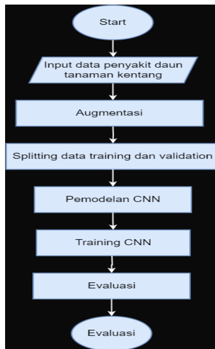
Gambar 3. 2 Pemodelan CNN
