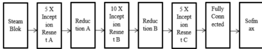
Gambar 2. 7 Skema Inception Resnet-V2 (Sumber : Ejournal Universitas majalengka )
