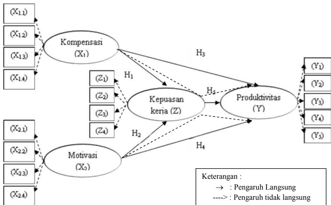
Gambar 2.3 Kerangka Konseptual
