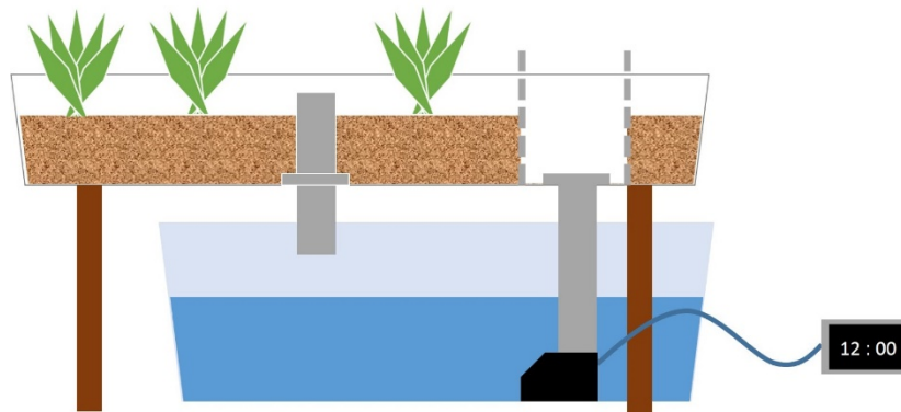
Gambar 2.2 Hidroponik Sistem Pasang Surut
