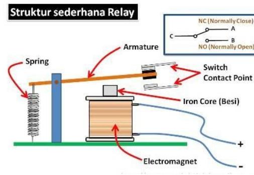
Gambar 2.5 Struktur Sederhana Relay (Sumber : www.produksielektronik.com )
