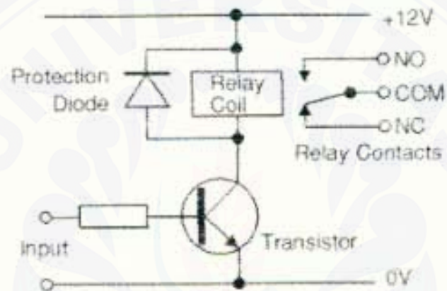
Gambar 2.15 Simbol Rangkaian Relé
