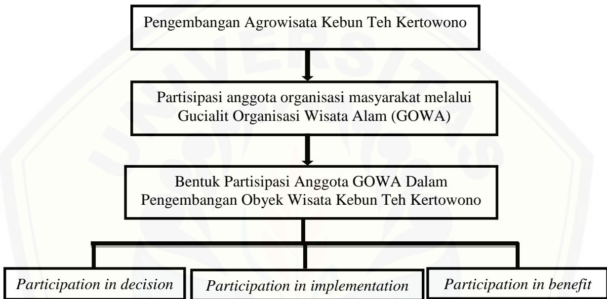
Gambar 2.2 Kerangka Berpikir
