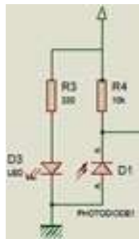
Gambar 2.8 Rangkaian Dasar Photodiode
