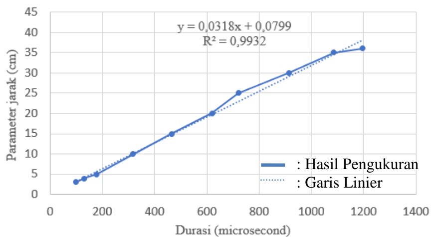
Gambar 3.17 Grafik Hasil Kalibrasi Sensor
