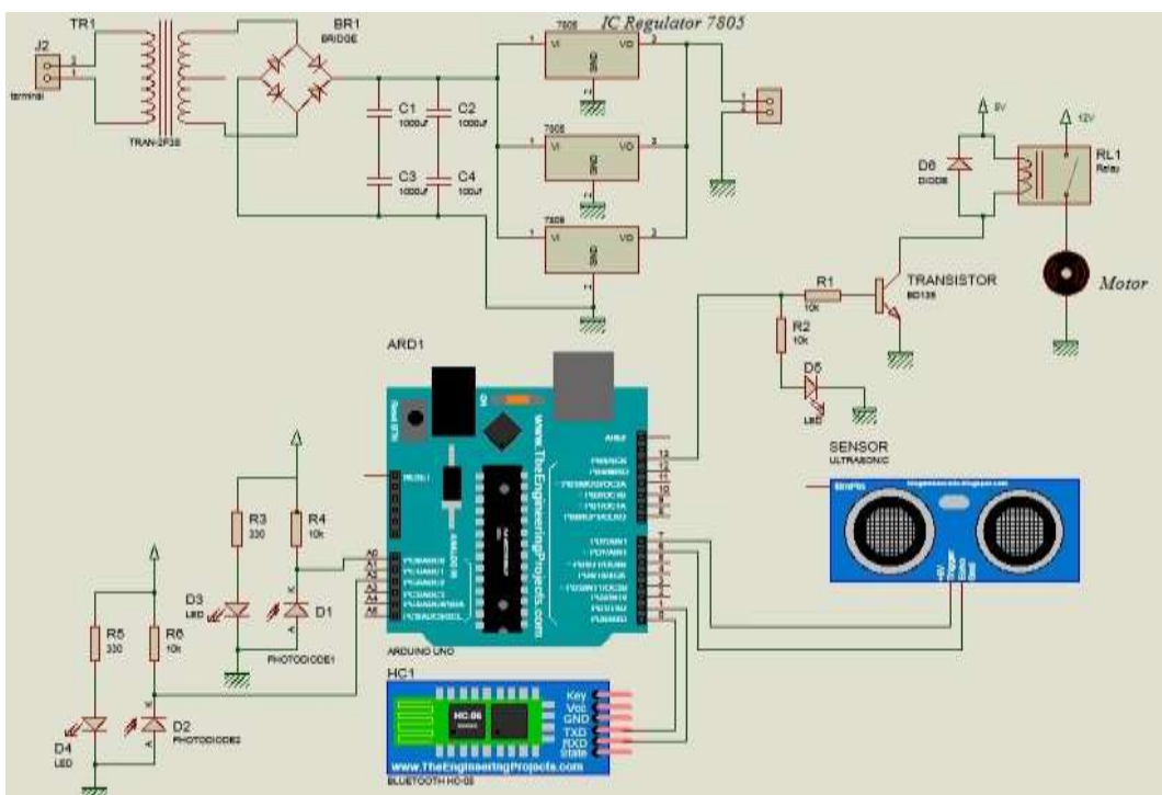
Gambar 3.10 Rangkaian Keseluruhan
