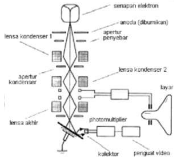
Gambar 2.1 Diagram skematik cara kerja SEM (Sumber: Anggraeni, 2008)
