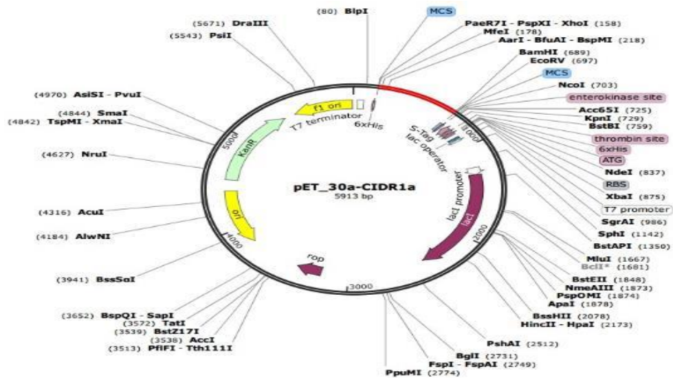
Gambar 3. Map DNA Rekombinan pET-30a-CIDR1α.
