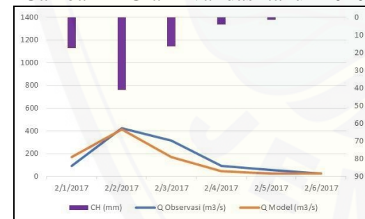
Gambar 13 Grafik validasi tahun 2017
