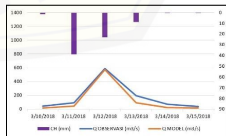
Gambar 21 Grafik puncak debit banjir skenario 1
