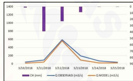
Gambar 25 Grafik puncak debit banjir skenario 3
