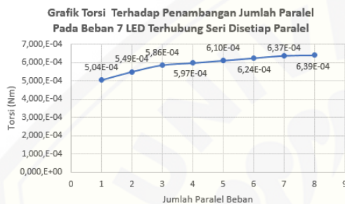
Gambar 16. Grafik Torsi Terhadap Penambahan Jumlah Paralel Pada Beban 7 LED Terhubung Seri Disetiap Paralel
