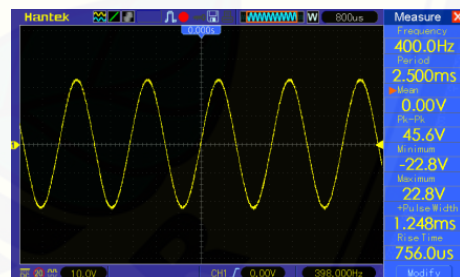
Gambar 11. Frekuensi Gelombang Luaran AC
