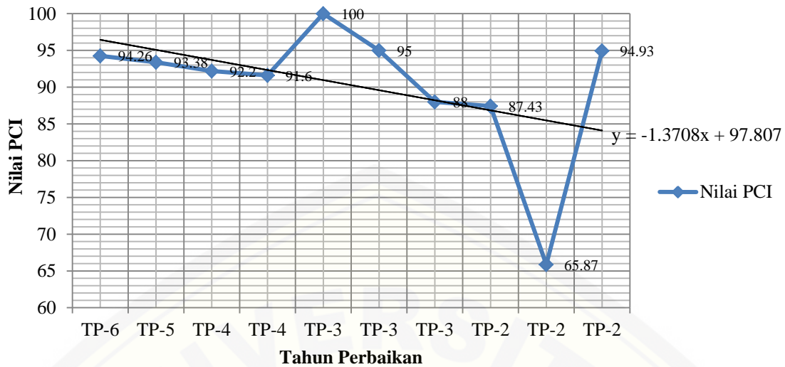
Gambar 2. Grafik hubungan tahun perbaikan dengan nilai PCI
