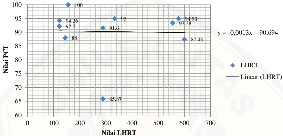
Gambar 3. Grafik hubungan nilai LHRT dengan nilai PCI
