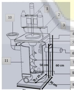
Gbr. 1 Desain Alat Starter Fermentor Stater Modified Cassava Flour (MOCAF) dengan Fuzzy
