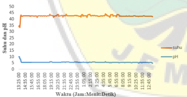
Gbr. 14 Grafik Pembacaan Sensor Suhu DS18B20 dan Sensor pH Fermentasi Stater MOCAF
