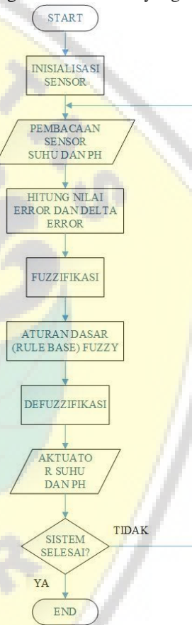
Gbr. 2 Diagram Alir Alat Stater Modified Cassava Flour (MOCAF) dengan Fuzzy
