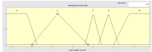
Gbr. 8 Fungsi Keanggotaan Error Input pH
