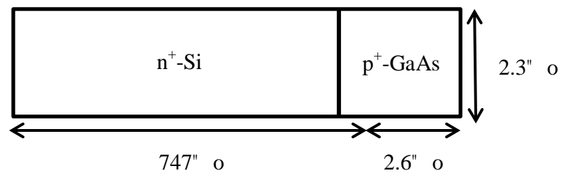
Gambar 3.3 Geometri struktur 2D dari p + -GaAs/n + -Si heterojunction dengan panjang 747.6" x 2.3" o
