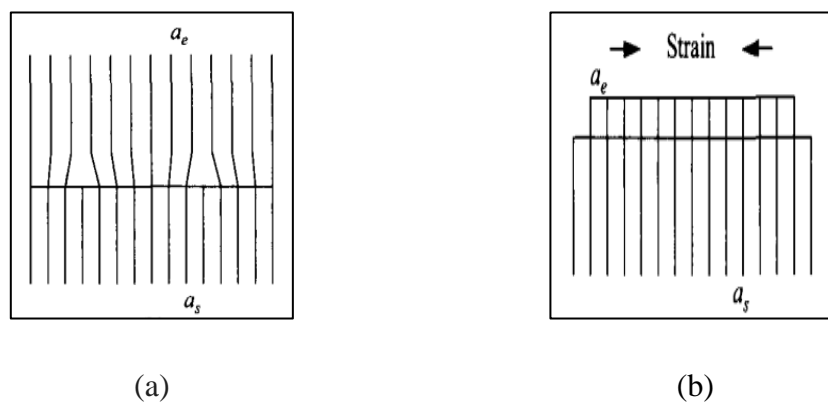
Gambar 2.4 Dua material dengan ketidakcocokan konstanta kisi dan (a) ketebalan lapisan sangat tebal, memiliki dislokasi antar muka (b) ketebalan lapisan tipis, peregangan terjadi sehingga tidak terjadi dislokasi (Sze, 2007).
