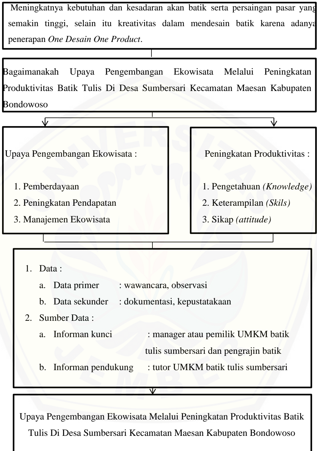
Gambar 3.1 rancangan penelitian
