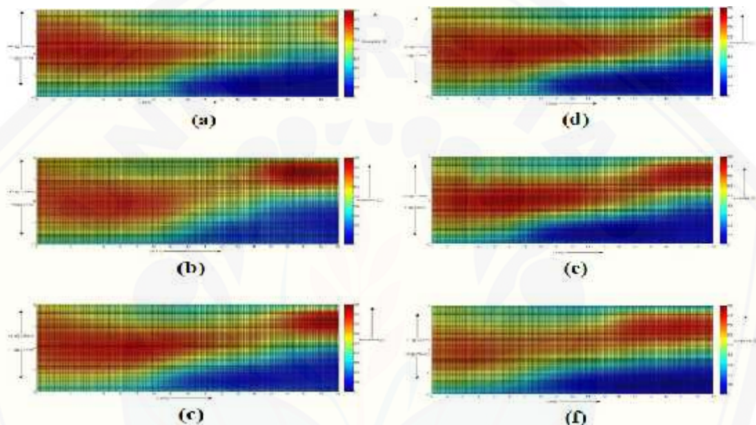
Gambar 2.6. Distribusi temperatur api difusi counterflow flame (Toko dkk, tanpa tahun)
