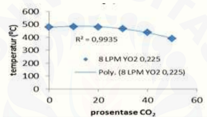
Gambar. 2.7 Grafik hubungan prosentase CO_2 pada bahan bakar terhadap temperatur (Toko dkk, tanpa tahun)
