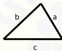
Segitiga Lancip
