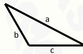
Segitiga Tumpul
