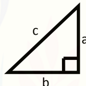
Segitiga Siku-siku
