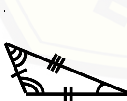
Segitiga sembarang
