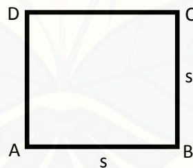
Gambar 2.2 Persegi
